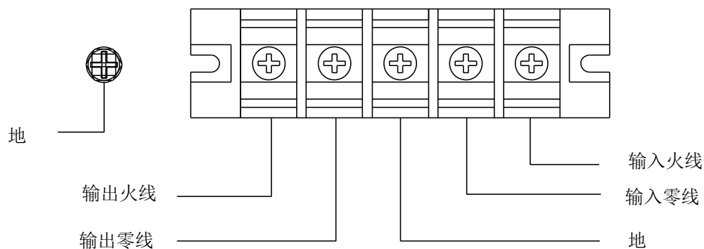
端子台接线图
